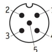
Ansicht Stiftkontakt
